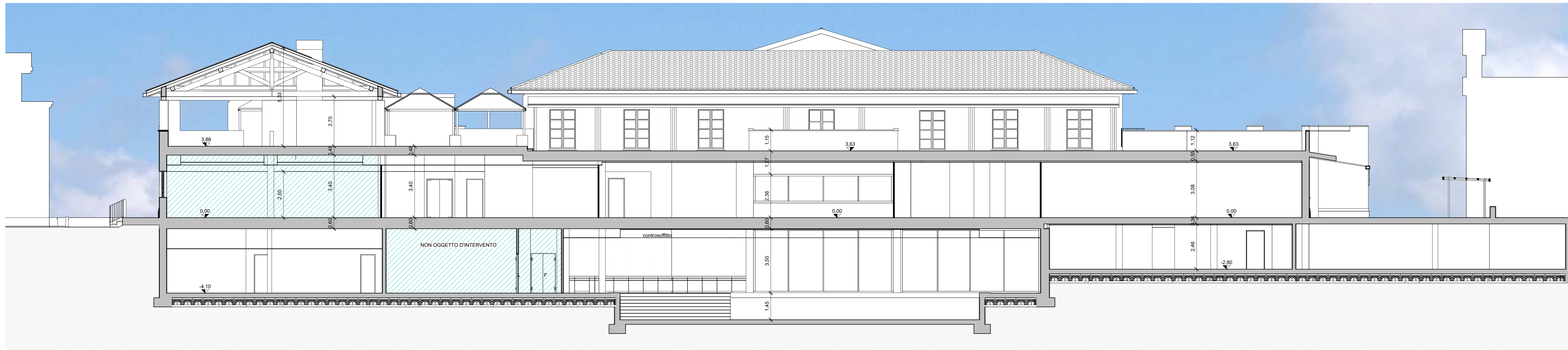
Sezione F Stato di fatto
